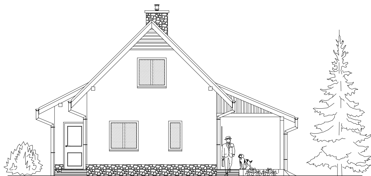
ELEWACJA FRONTOWA
