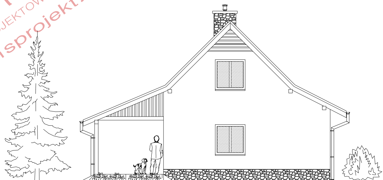
ELEWACJA TYLNA
